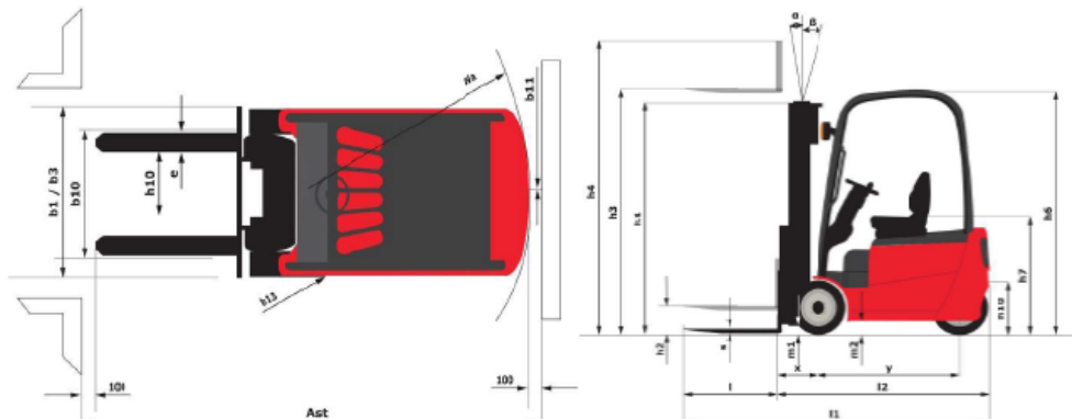
ME 430 - Disegno quotato
